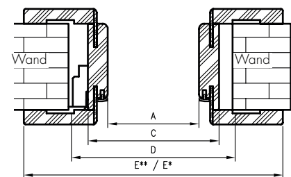
Horizontalschnitt OR/ORC
