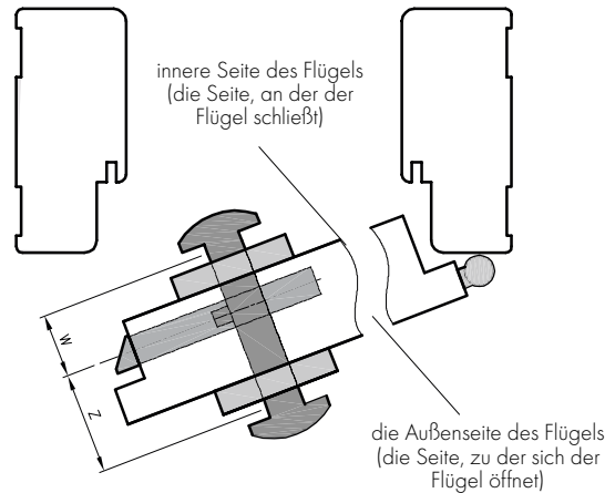
Abb. Auswahl der Größe des Zylinders mit Drehknopf
