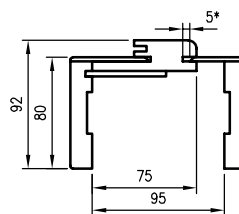
Schnitt ORB 075
