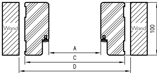
Maßen für einflügelige Türen
