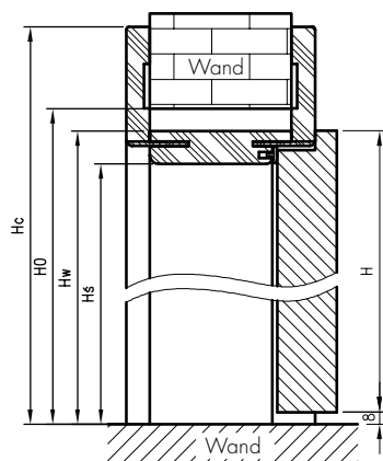
Vertikalschnitt OR
