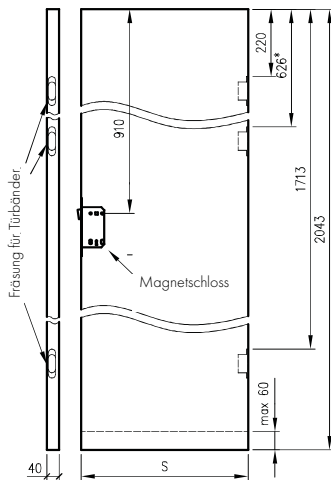
Türflügel ohne Falz
