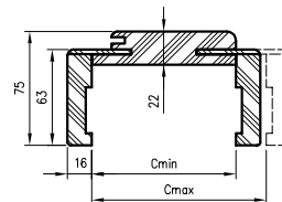
Schnitt OR/ORC mit Winkel T63
