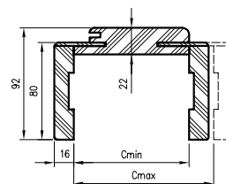
Schnitt OR/ORC mit Winkel T80
