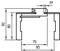
Schnitt ORB 075
