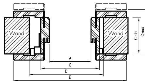
Horizontalschnitt ORB
