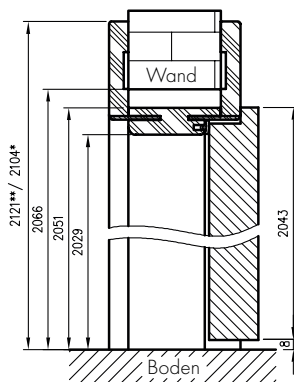
Vertikalschnitt eines Türflügels mit Falz mit OR
