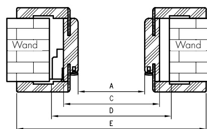
Horizontalschnitt OR
