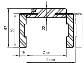
Schnitt OR/ORC-Profil mit Winkel T80
