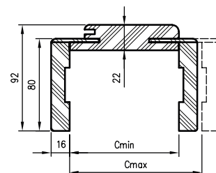
Horizontalschnitt OR
